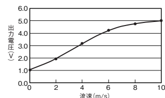
形D6F-W01A1
