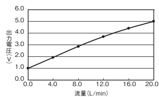
形D6F-20A5-000
