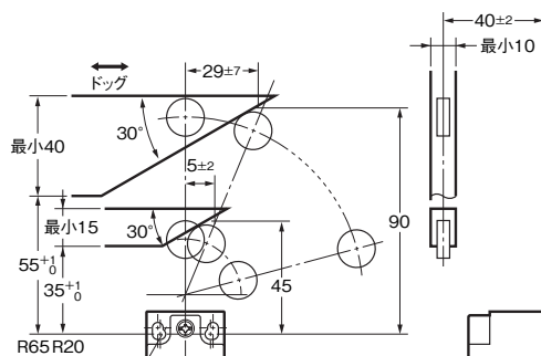
ローラ・プランジャ形 (形D4N-□□32)
