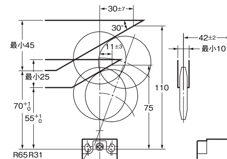
可変ローラ・レバー形・フォームロックタイプ (金属レバー、ゴムローラ) (形D4N-□□2H) (参考値)
