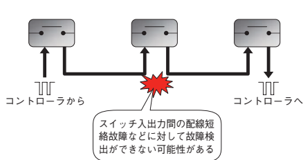
メカスイッチタイプのシリーズ接続時
