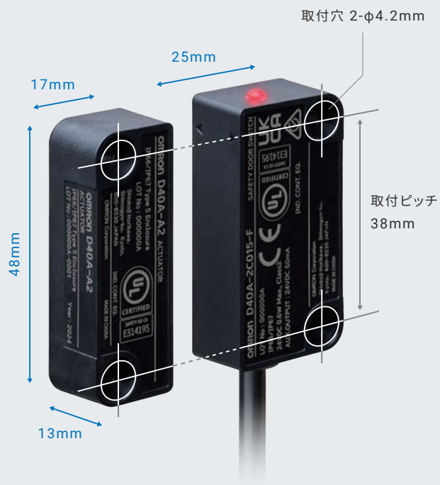
D40A-2原寸大
