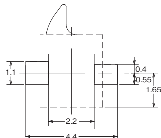
プリント基板パッド寸法図(参考) (TOP VIEW)
