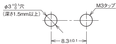
取り付け穴加工寸法 (参考)
