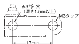
取り付け穴加工寸法(参考)
