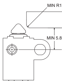
M3ねじ取り付け
