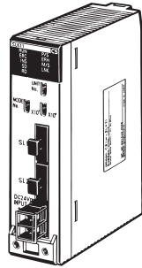
●H-PCF光タイプ 形CS1W-SLK11
