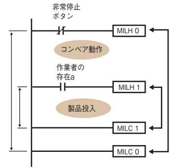
●CX-Programmer画面
