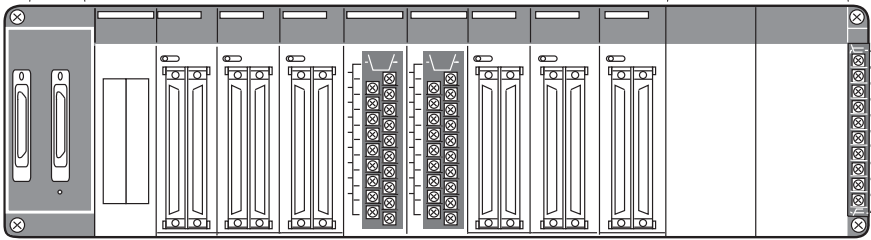
■増設ケーブル接続コネクタ 増設ユニット/Fケーブルを装着する。
