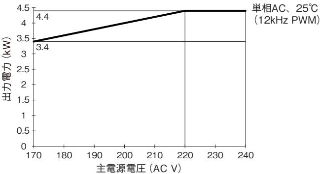
単相入力電圧時の電力出力ディレーティング (形CK3A-G320Lのみ)
