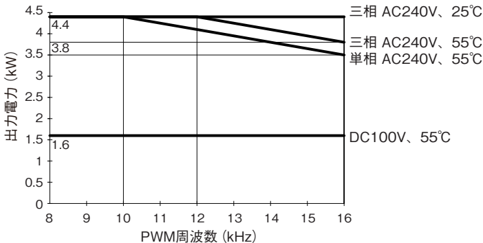
PWM周波数による電力出力ディレーティング (形CK3A-G320Lのみ)
