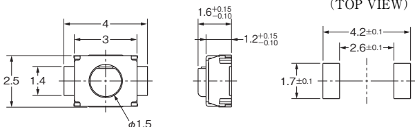
プリント基板パッド寸法例 (TOP VIEW)
