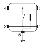
端子配置/内部接続図 (TOP VIEW)
