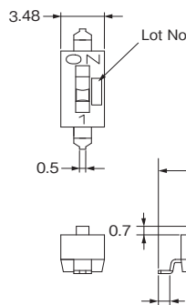
1極スイッチ外形寸法図
