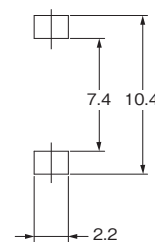
1極PCBレイアウト
