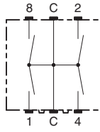
上面操作 3×3端子
