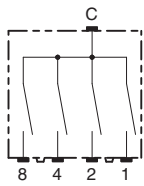
上面操作 4×1端子
