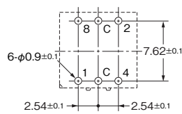
上面操作 3×3端子
