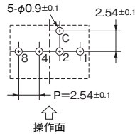
側面操作 4×1端子
