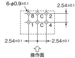
側面操作 3×3端子
