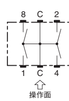
側面操作 3×3端子
