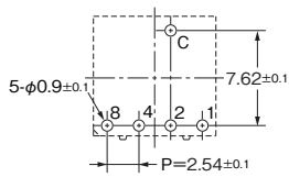
上面操作 4×1端子
