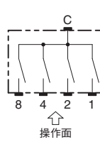
側面操作 4×1端子
