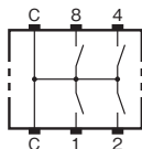
内部接続図 (TOP VIEW)
