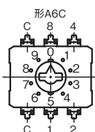
端子配置
