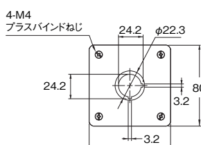
コントロールボックス 形A22NZ-A-B101 形A22NZ-A-B101Y
