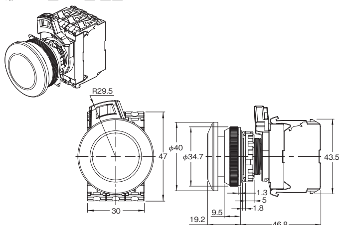
きのこ形(金属ベゼル) 形A30N□-MM□-□□A-G
