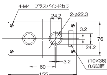
コントロールボックス(2穴) 形A22NZ-A-B102
