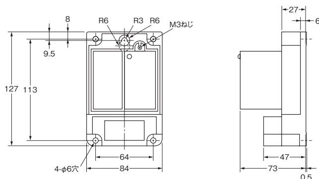
取り付け穴加工寸法
