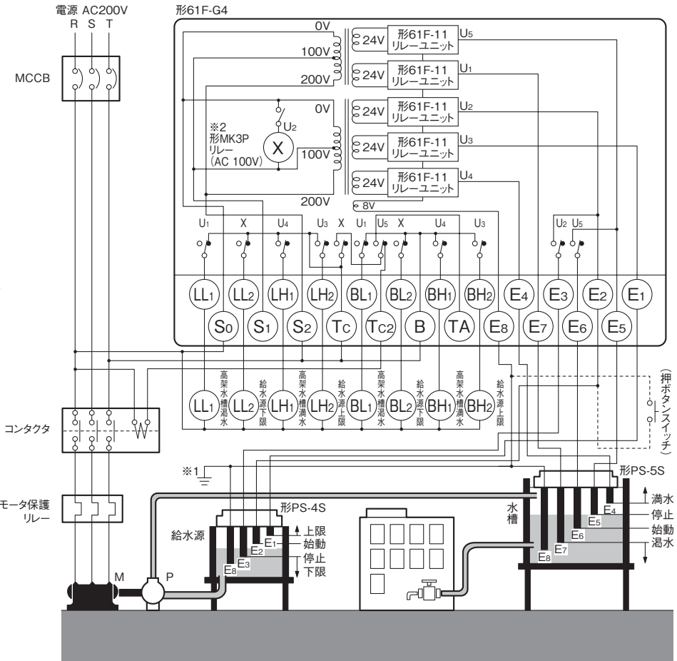
給水源の水位表示と湯水によるポンプの空転防止および高架水槽の水位表示を兼ねた給水の自動運転
