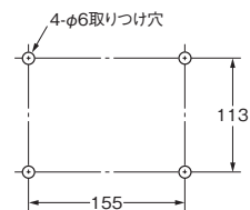
取り付け穴加工寸法
