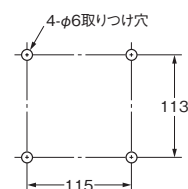
取り付け穴加工寸法
