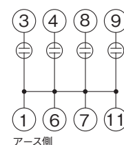
形61F-04B 電極接続端子側
