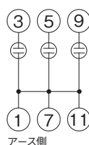
形61F-03B 電極接続端子側
