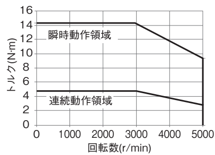
・形R88M-1AL1K530C
