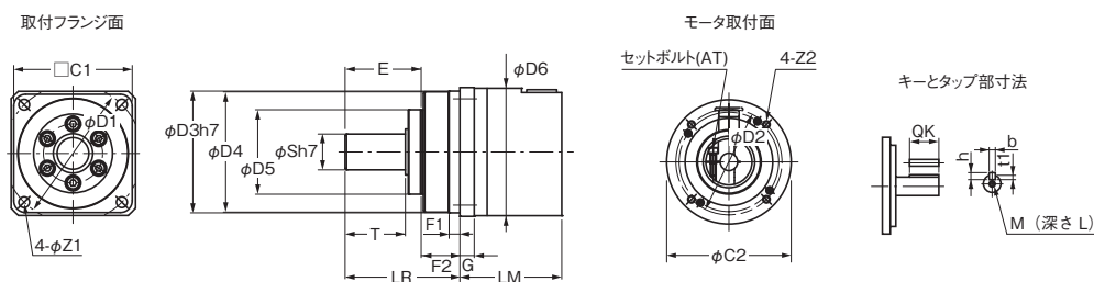
外形図2
