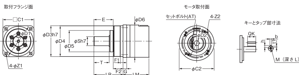
外形図2
