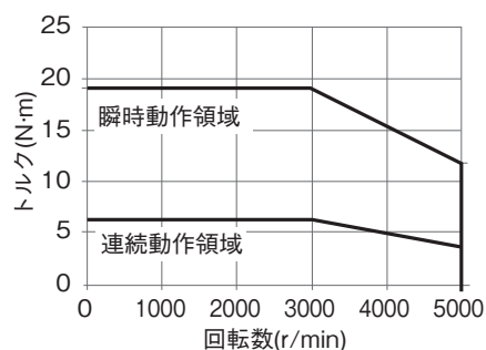
・形R88M-1AL2K030C
