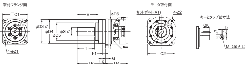
外形図2
