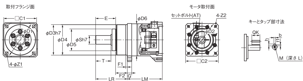
外形図2
