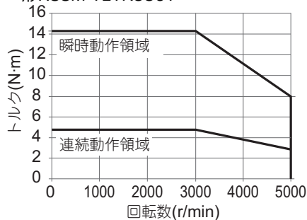
・形R88M-1L4K030T
