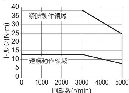
・形R88M-1L4K030C
