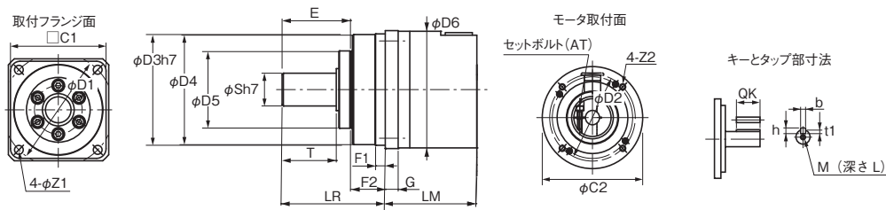
外形図2
