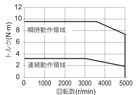
・形R88M-1L1K030T
