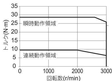
・形R88M-1M2K020C
