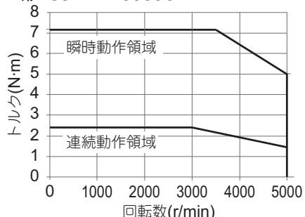
・形R88M-1L2K030C
