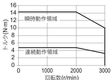
・形R88M-1M3K020T
