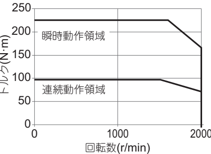
・ 形R88M-1M15K015C
