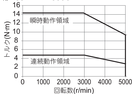
・形R88M-1L4K030C
