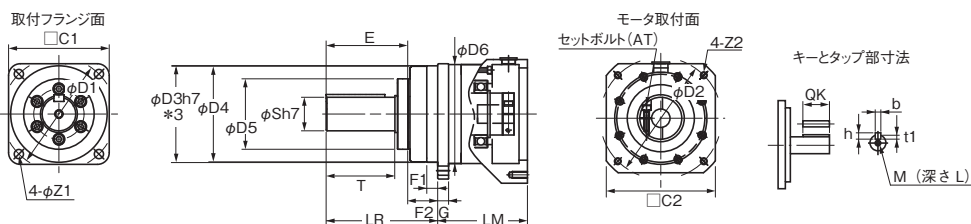
外形図1
