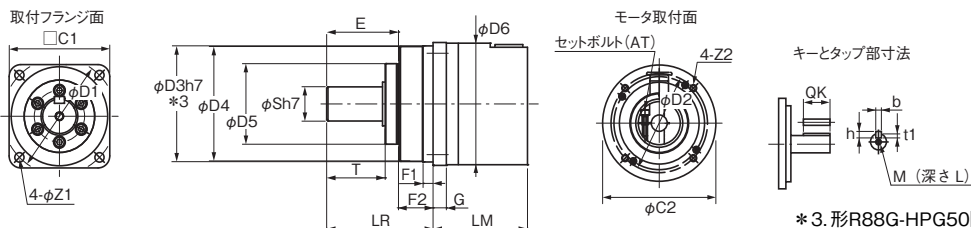
外形図2
