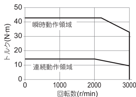
・形R88M-1M3K020C
