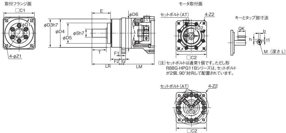
外形図2
