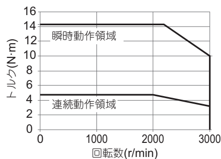
・形R88M-1M1K020C
