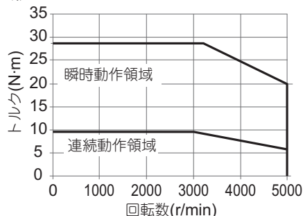
・形R88M-1L3K030C
