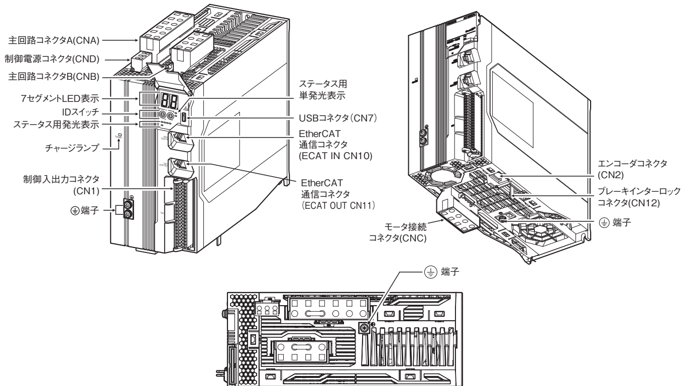
上面図
