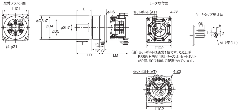
外形図2
