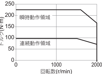
・形R88M-1M15K015C
