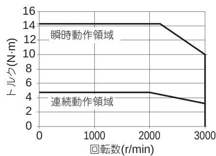
・形R88M-1M1K020C
