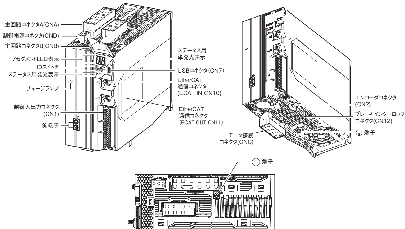
上面図
