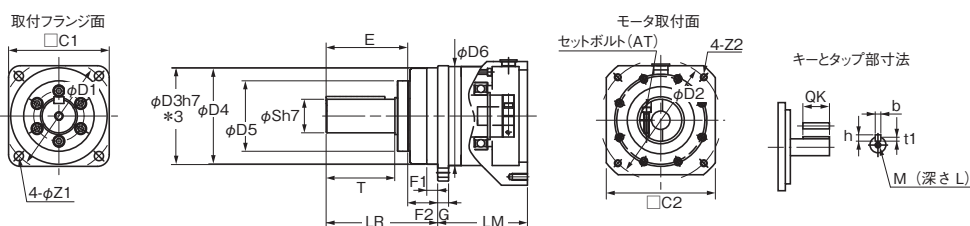
外形図1
