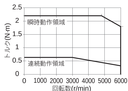
・形R88M-1M20030T
