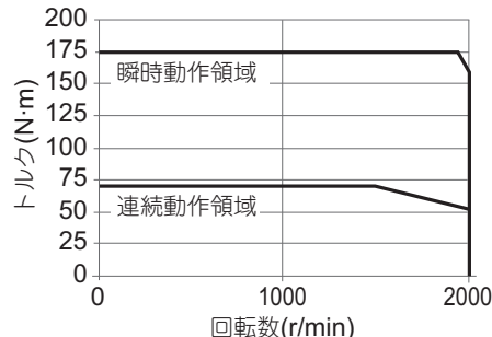
・形R88M-1M11K015C
