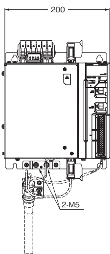
外形寸法
