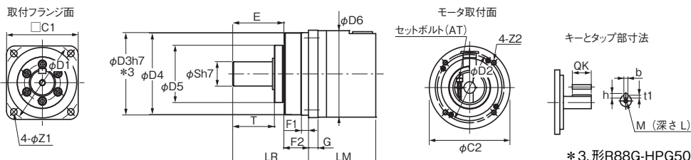
外形図2
