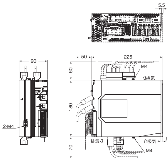
外形寸法
