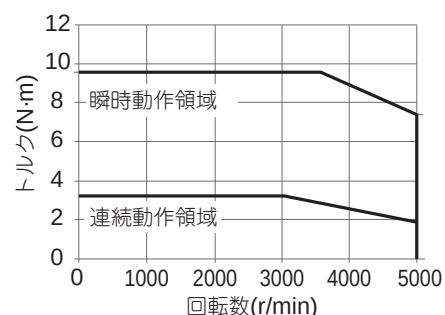
・形R88M-1L1K030T
