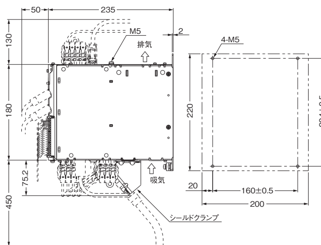
取付寸法
