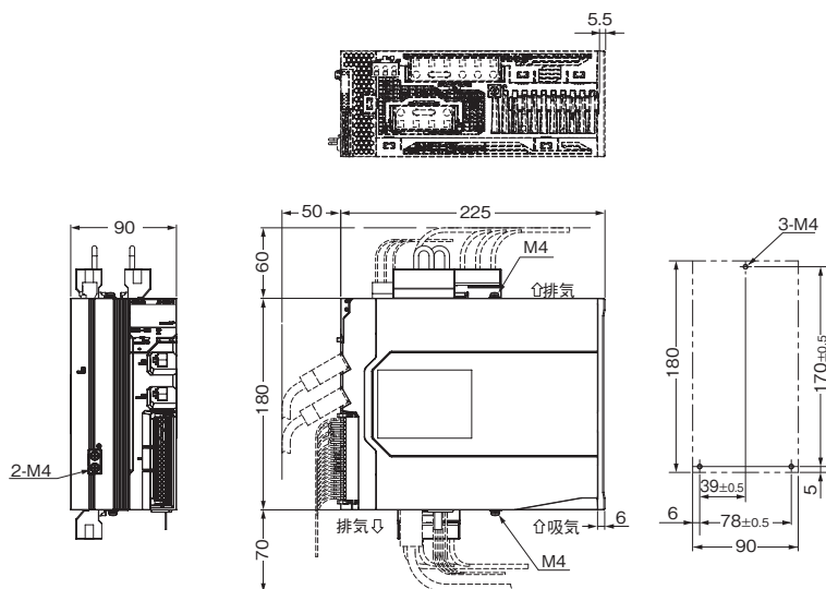
取付寸法
