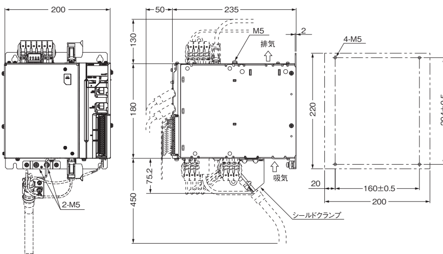
取付寸法
