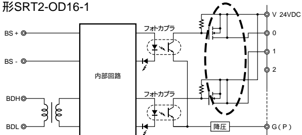
形SRT2-OD16-1
