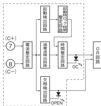
図10. 形SE静止形モータ・リレー(瞬時タイプ)内部ブロック図 反限時タイプにおける[ ]の部分の下図のようになります。
