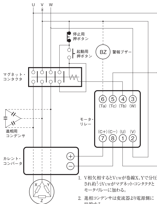
図7. 欠相時の電圧降下、進相コンデンサの位置
