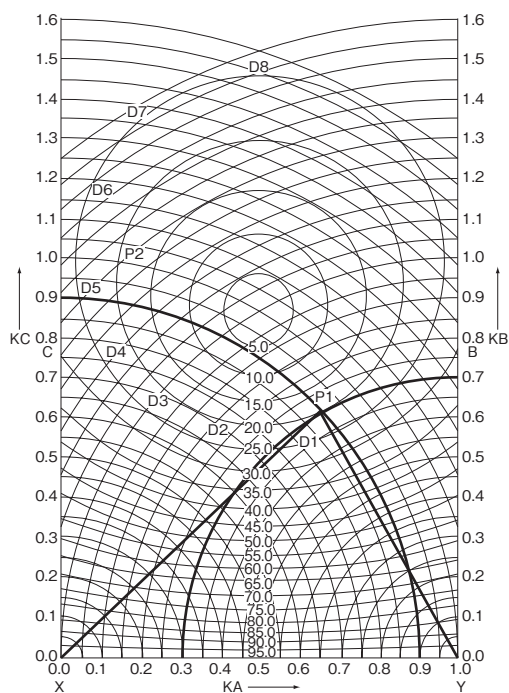
図18. 三相電流、電圧の不平衡率計算図表
