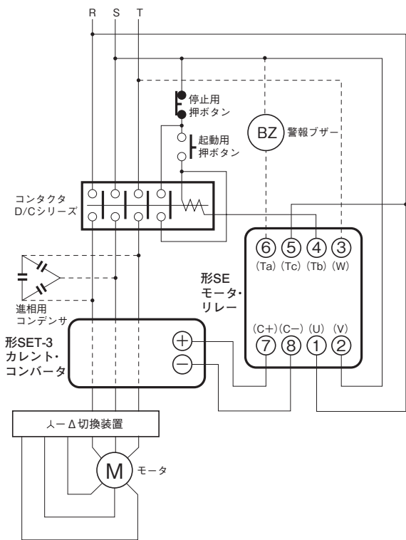
図17.(a) \Delta - \Delta 起動モータの場合の外部接続
