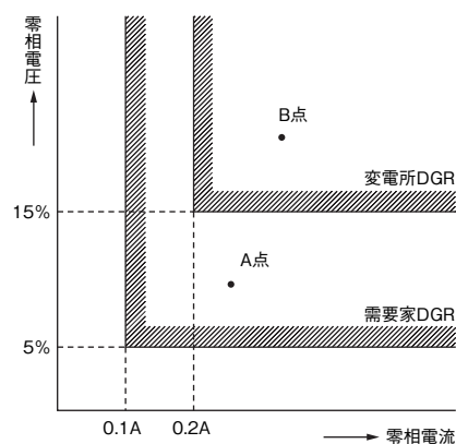
図3. DGRの感度協調例
