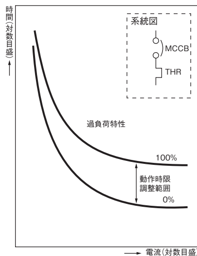
熱動形継電器保護協調曲線
