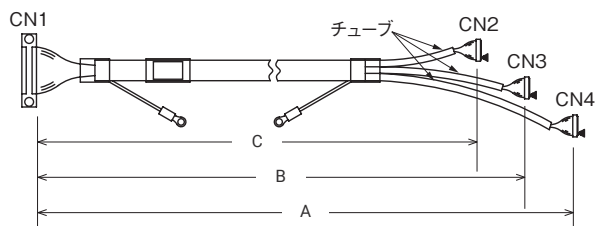
コネクタピン配置図 (コネクタかん合面より)
