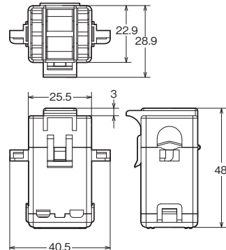
CT貫通穴内径寸法
