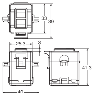
CT貫通穴内径寸法
