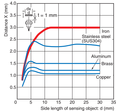
E2EQ-X3D1(-M1(T)GJ)
