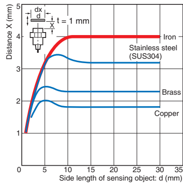
E2EQ-X3D1(-M1(T)GJ)
