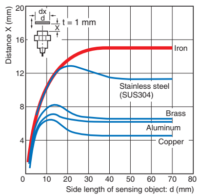
E2EQ-X10D1(-M1(T)GJ)
