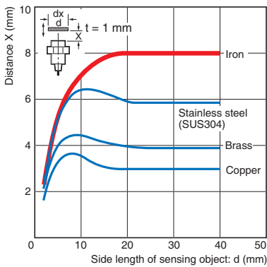
E2EQ-X7D1(-M1(T)GJ)
