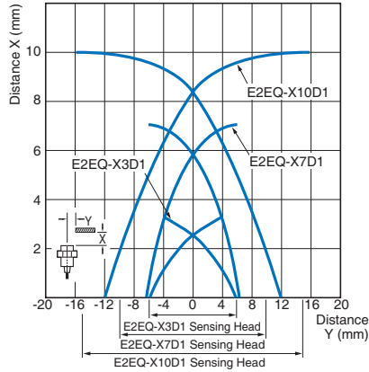
E2EQ-X□D□(-M1(T)GJ)
