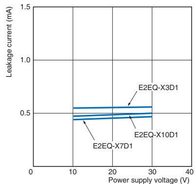
E2EQ-X□D
