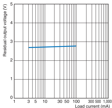
E2EQ-X□D□(-M1(T)GJ)
