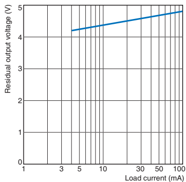
E2EQ-X□X□(-M1(T)J)
